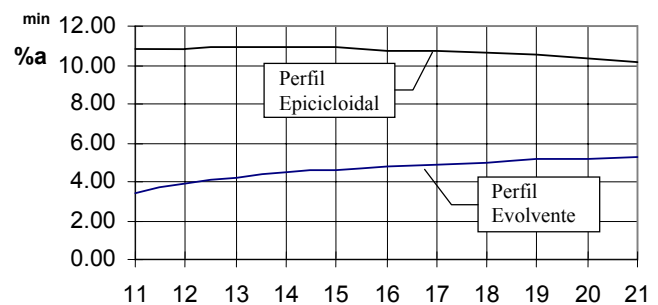
Fig. 7. Variación de la distancia entre centros vs Z
