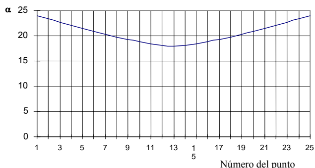
Fig. 8. Ángulo de presión ( \alpha ) vs punto de la línea de engranaje en el perfil epicicloidal alargado.
