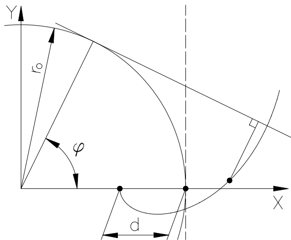
Fig. 2. Curva evolvente de círculo.
