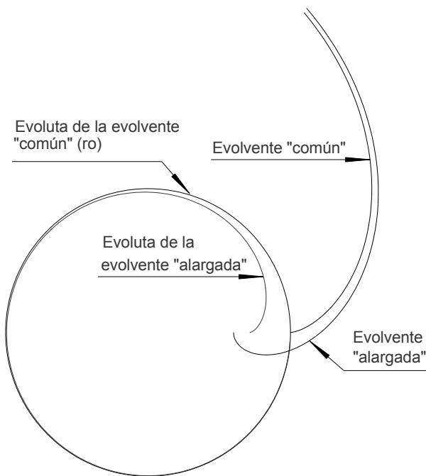
Fig.4. Comparación entre las evolventes.
