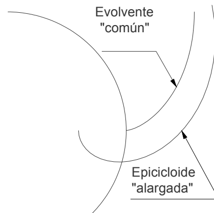
Fig.6. Comparación entre la epicicloide "alargada" y la evolvente "común".
