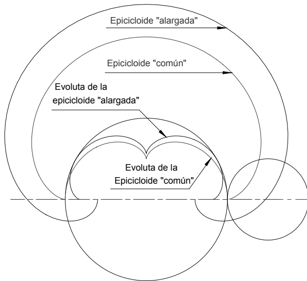
Fig.3. Comparación entre las epicicloides.
