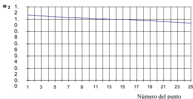
Fig. 9. Velocidad angular ( \omega_2 ) vs punto de la línea de engranaje en el perfil epicicloidal alargado.
