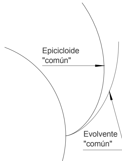
Fig.5. Comparación entre la epicicloide y evolvente comunes.
