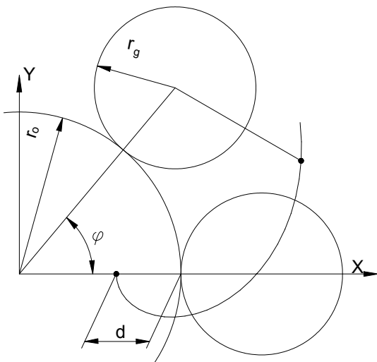
Fig 1. Curva epicicloidal.
