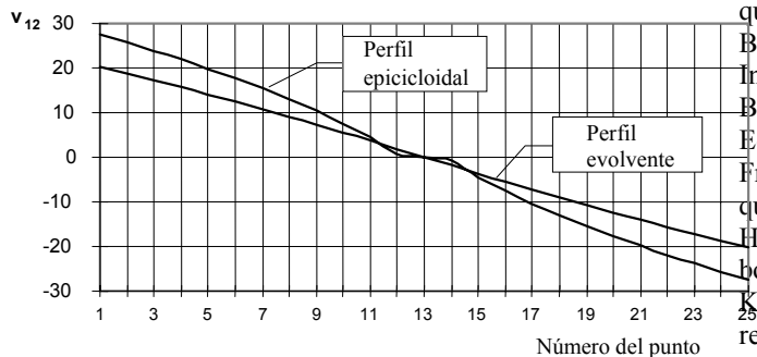
Fig. 10. Velocidad de deslizamiento relativo ( v_{12} ) vs punto de la línea de engranaje.
