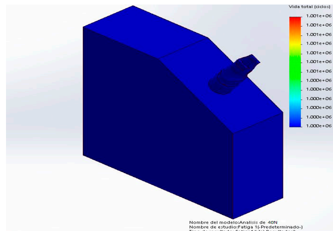
FIGURA 9. Ciclo de vida del implante dental y el hueso aplicando una carga de 40 N.
