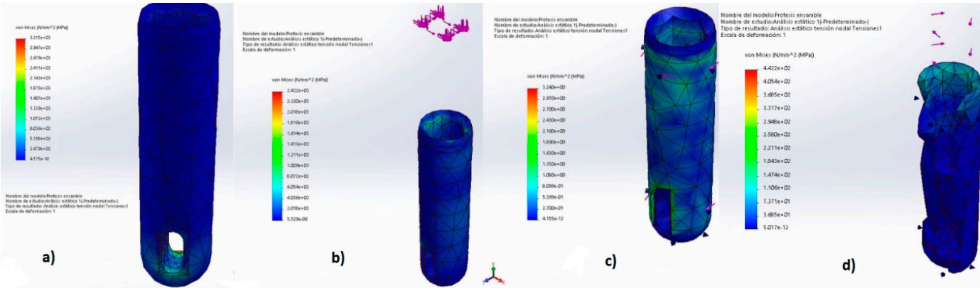
FIGURA 4. Distribución de Esfuerzos en el Cuerpo del Implante Cuando se le Aplican Cargas de: a) compresión, b) oblicua, c) torsional en el Cuerpo del Implante y d) torsional en el Tornillo de Fijación.
