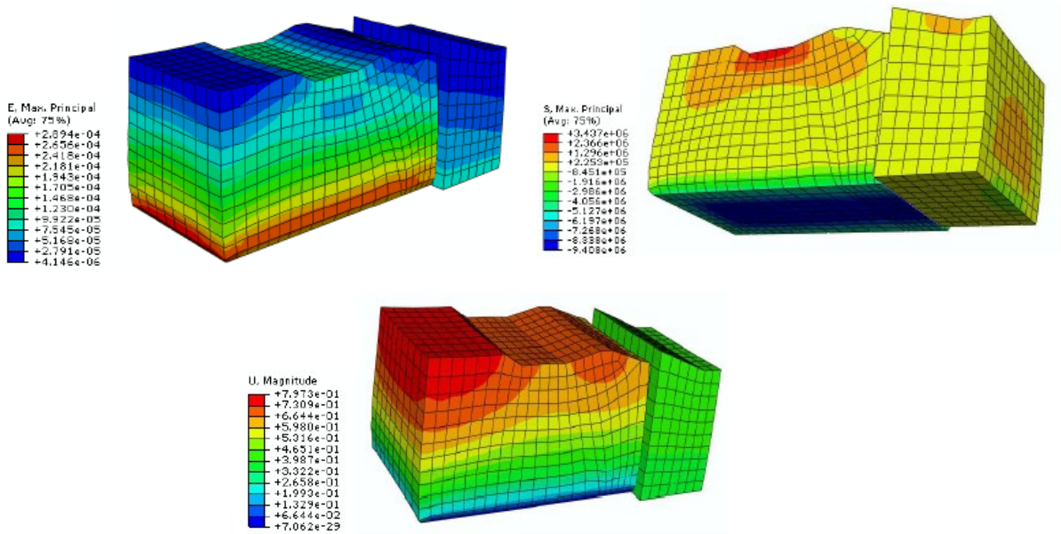
FIGURA 4. Desplazamientos, esfuerzos y deformaciones calculados para el modelo 1
